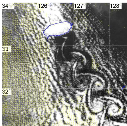
Вихревая дорожка Кармана к юго-востоку от о. Чеджу (Корея) по мультиспектральным данным спутника NOAA-15 за 8.01.2015 г. (Алексанин и др., 2016)
